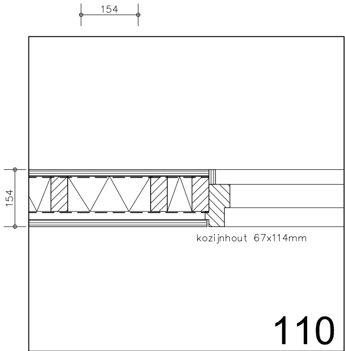
detail raamaansluiting
