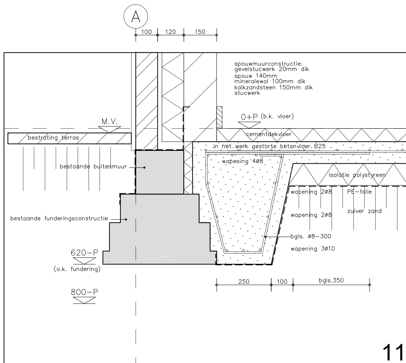
detail nieuwe fundering
