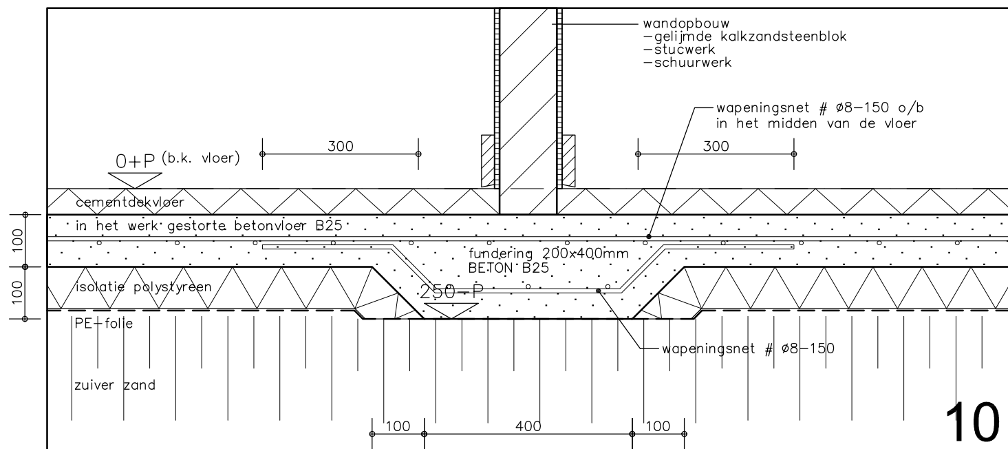
detail verzwaarde strook/ fundering
