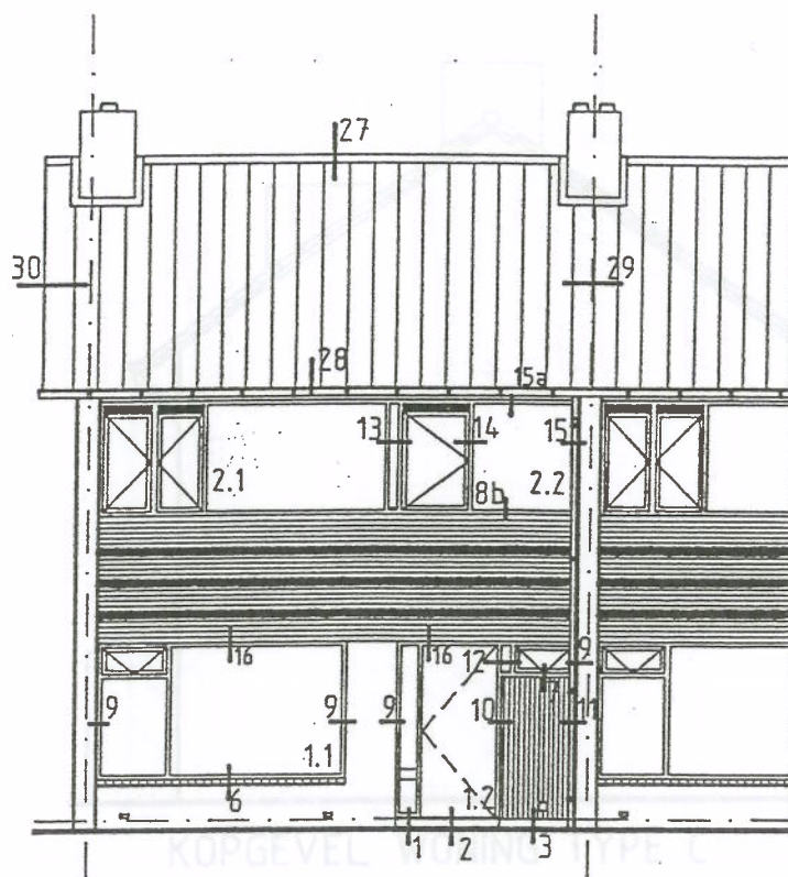
VOORGEVEL
