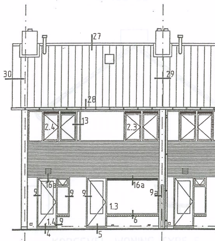
ACHTERGEVEL
