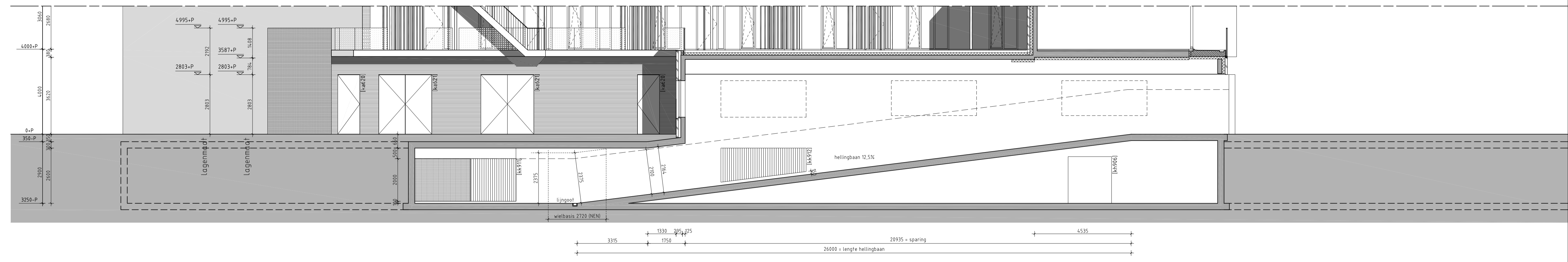
PARKEERGARAGE - doorsnede E1 - uitrit
