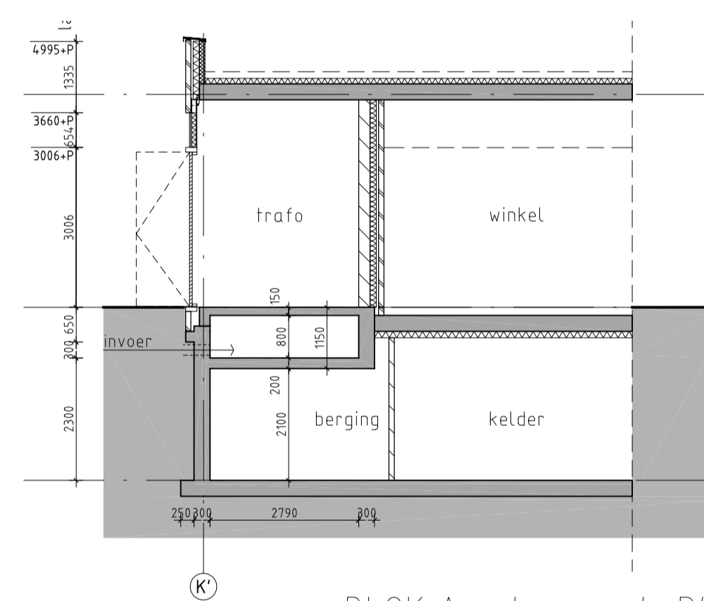
BLOK A - doorsnede D'
