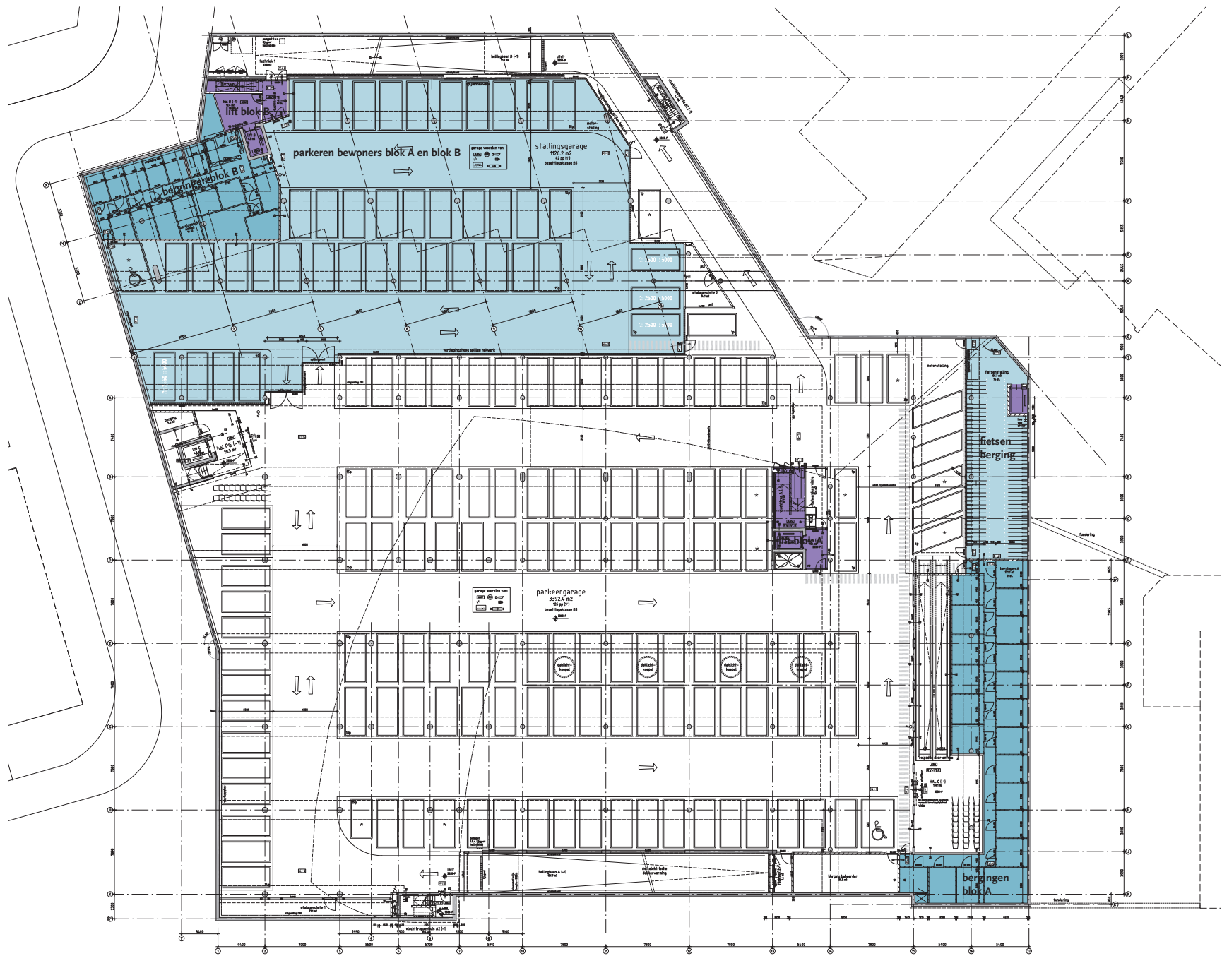
PARKEERGARAGE/BERGINGEN - plattegrond - 1:500
