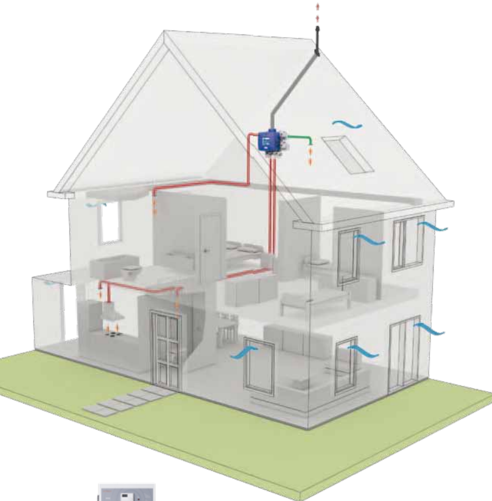
Ventilatie en zonwering in één
