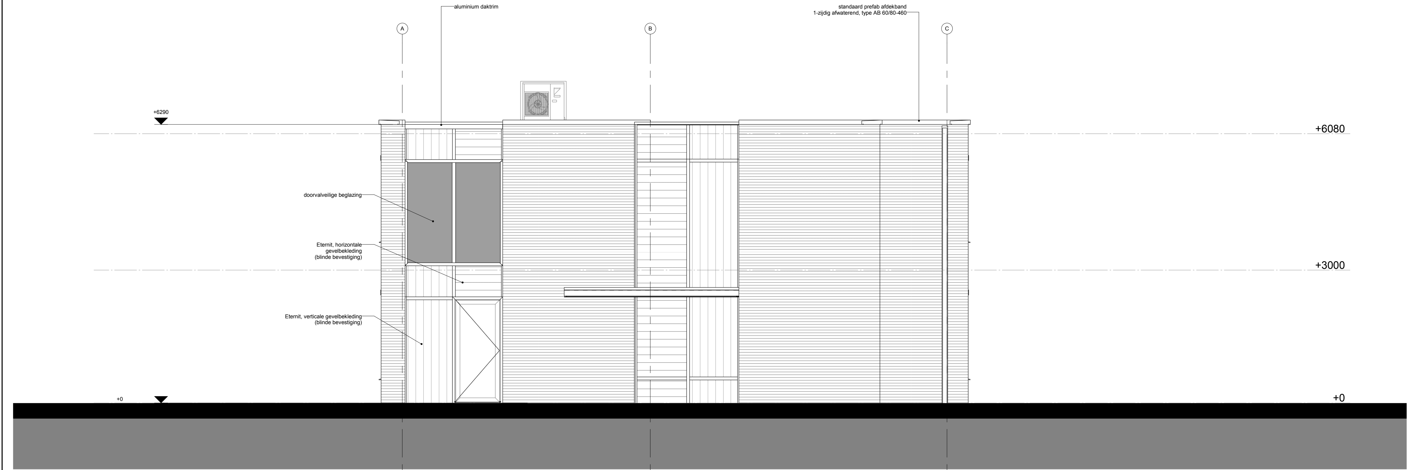
Zuidoostgevel
